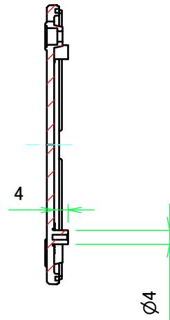
E-E ( 1 : 1.5 )
